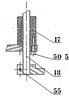
Section D-D
