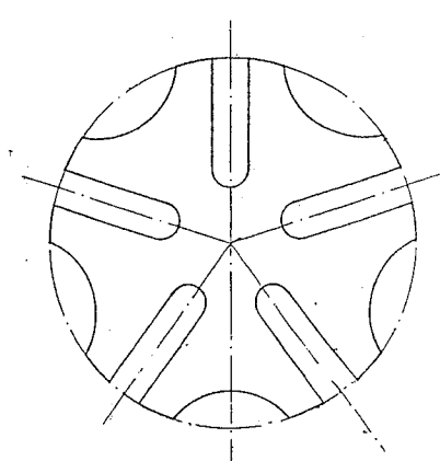
CROIX DE MALTE A 5 POSITIONS
